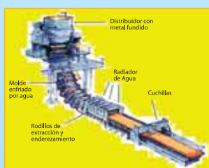
Un diagrama esquemático típico de la Fundición Continúa
