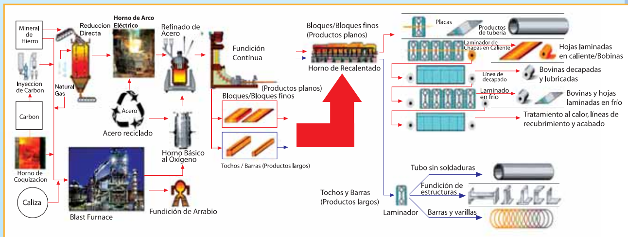
Proceso de producción de una Fundición Integrada (desde la Planta de Fundición hasta la Planta de Laminación)
